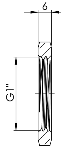
Ansicht / view A-A
